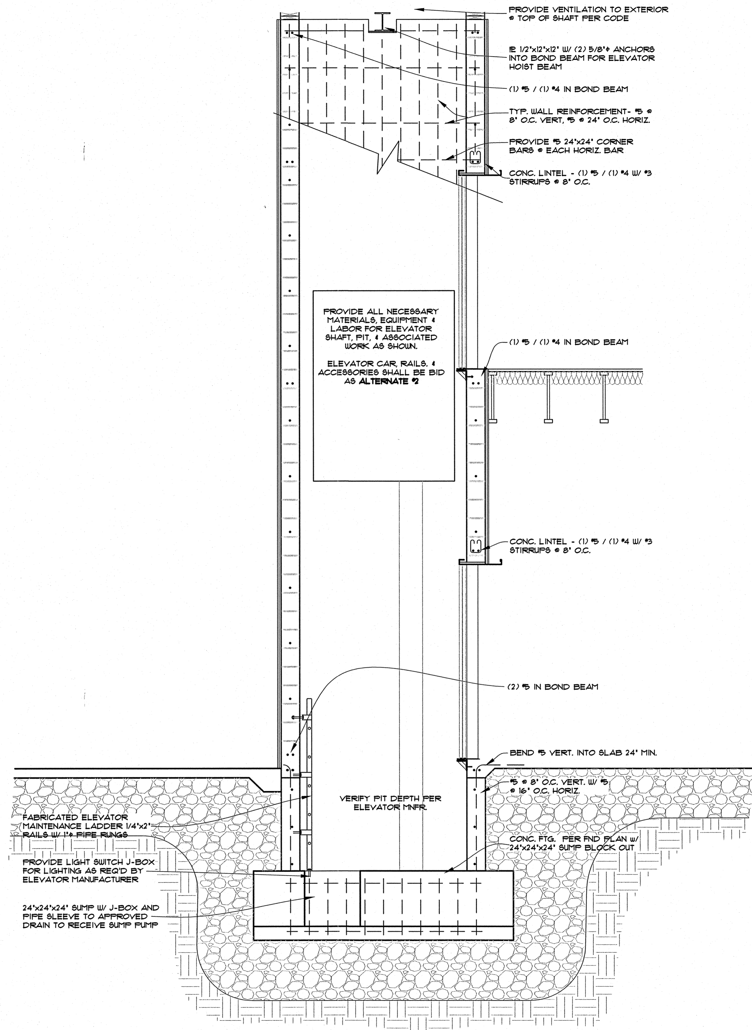
1 ELEVATOR SECTION A-4.1 SCALE: 1/2" = 1'-0"
